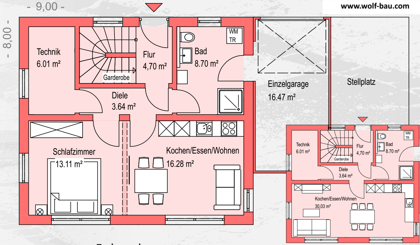
Erdgeschoss
