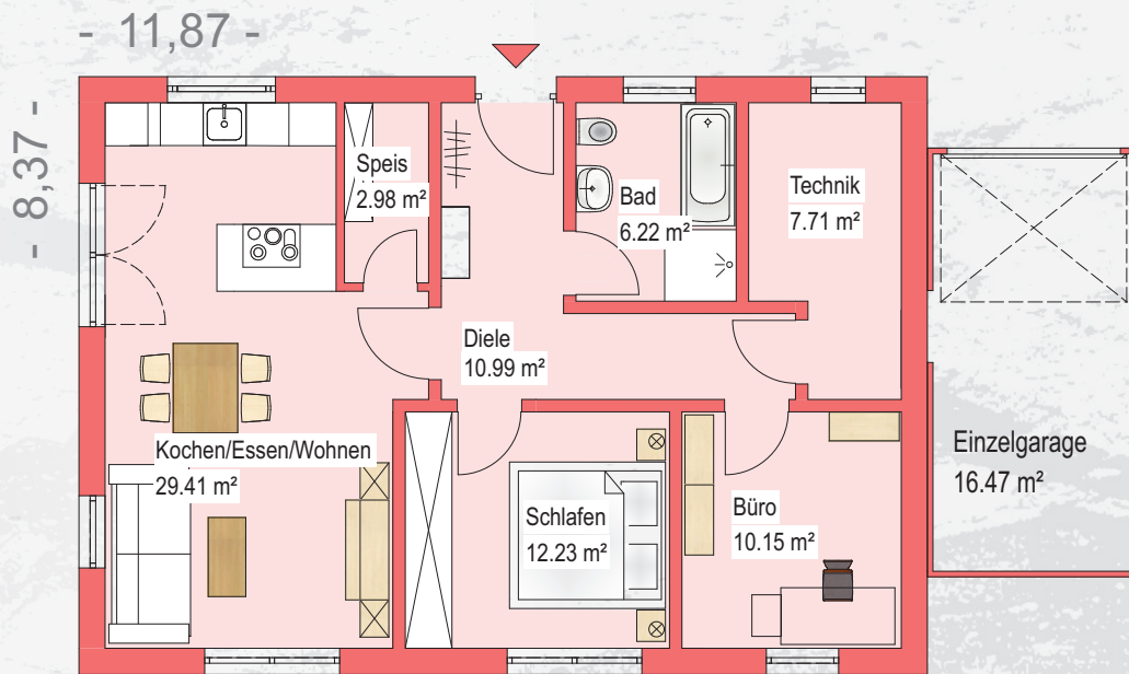
Grundriss Variante 1
