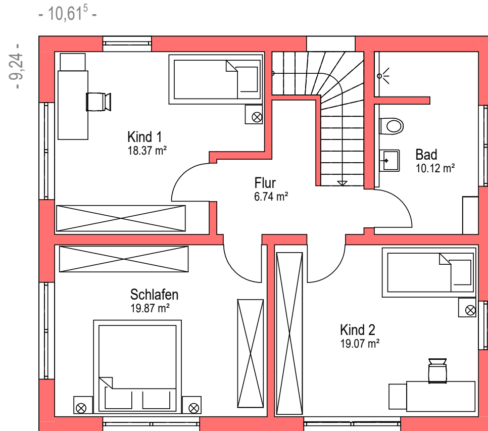
Obergeschoss
