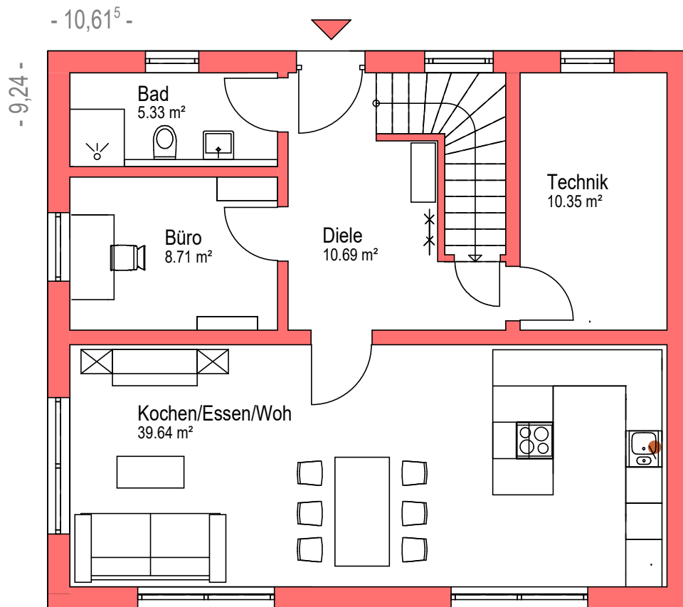
Erdgeschoss
