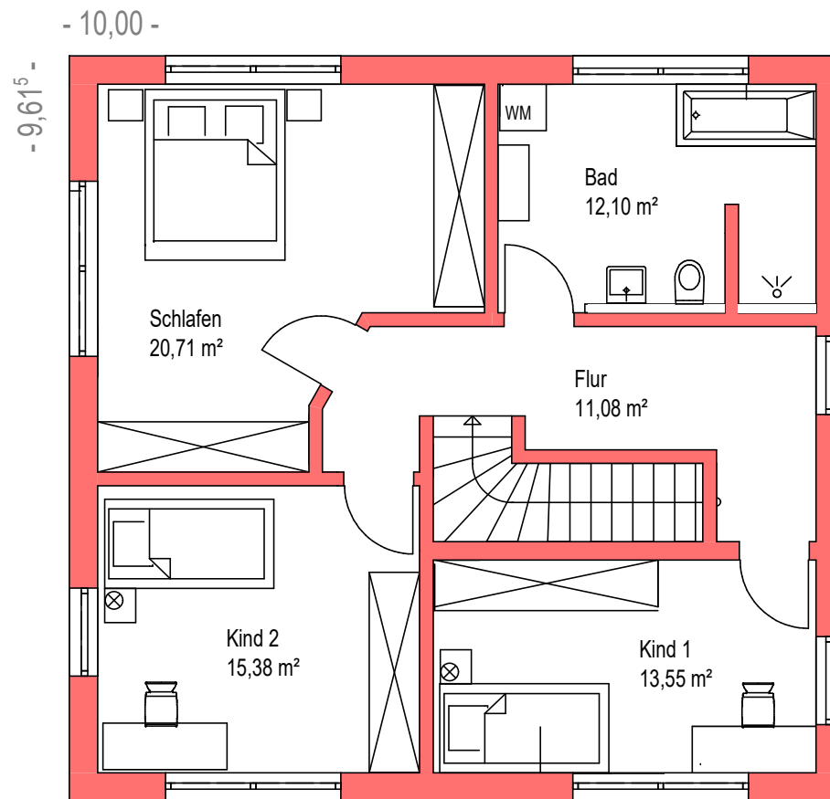
Obergeschoss
