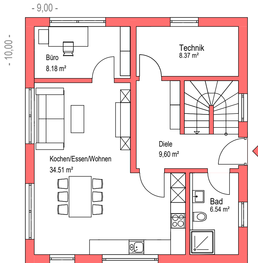
Erdgeschoss
