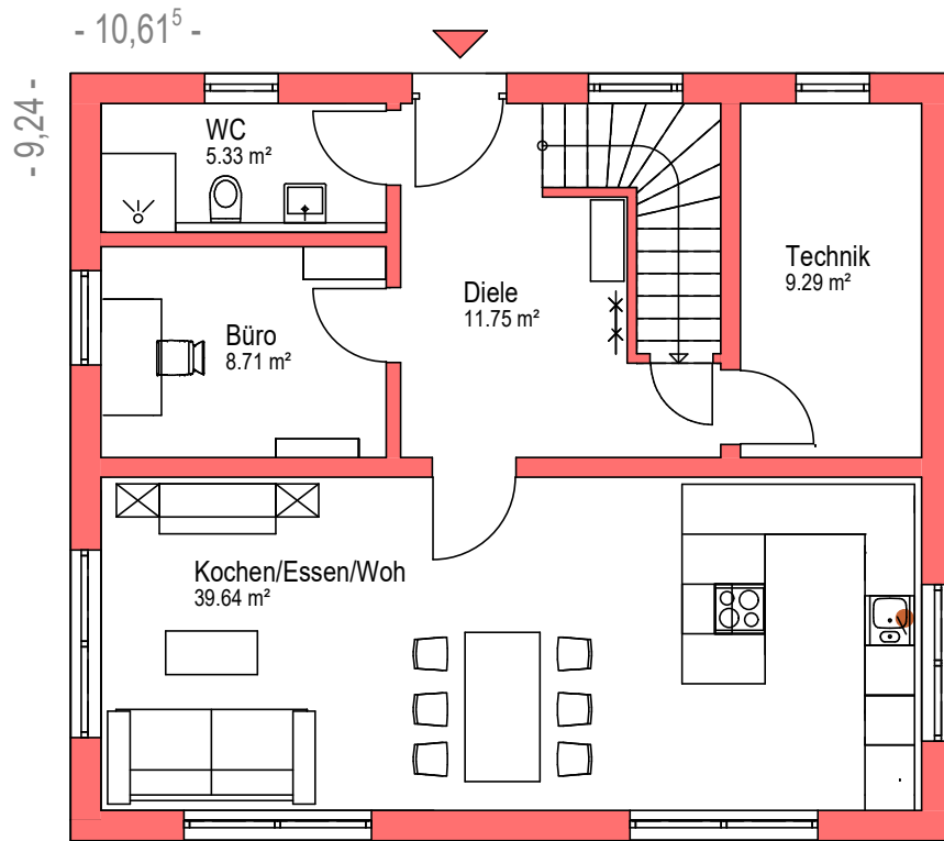
Erdgeschoss
