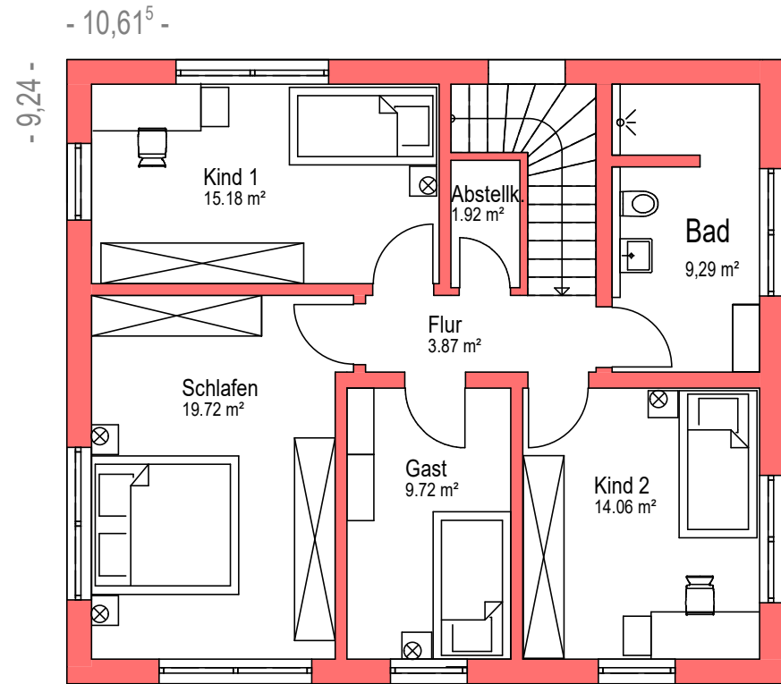
Obergeschoss
